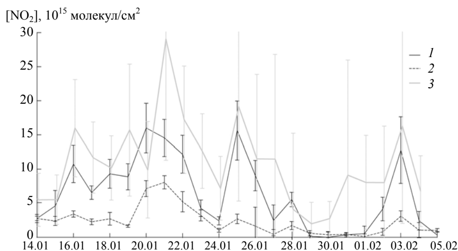
Рис. 3. Временной ряд среднедневных тропосферных содержаний NO 2 в районе Санкт-Петербурга в период с января по февраль 2016 г.: 1 — наземные измерения ИНОЗ, 2 — наземные измерения НИИФ, 3 — спутниковые измерения ОМІ
