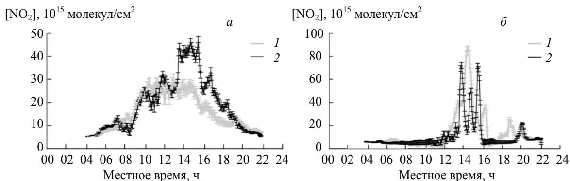
Рис. 4. Примеры дневных вариаций тропосферного содержания NO 2 в районе Санкт-Петербурга 17.05.2014 (а) и 25.05.2014 (б): 1 — наземные измерения ИНОЗ, 2 — наземные измерения НИИФ
